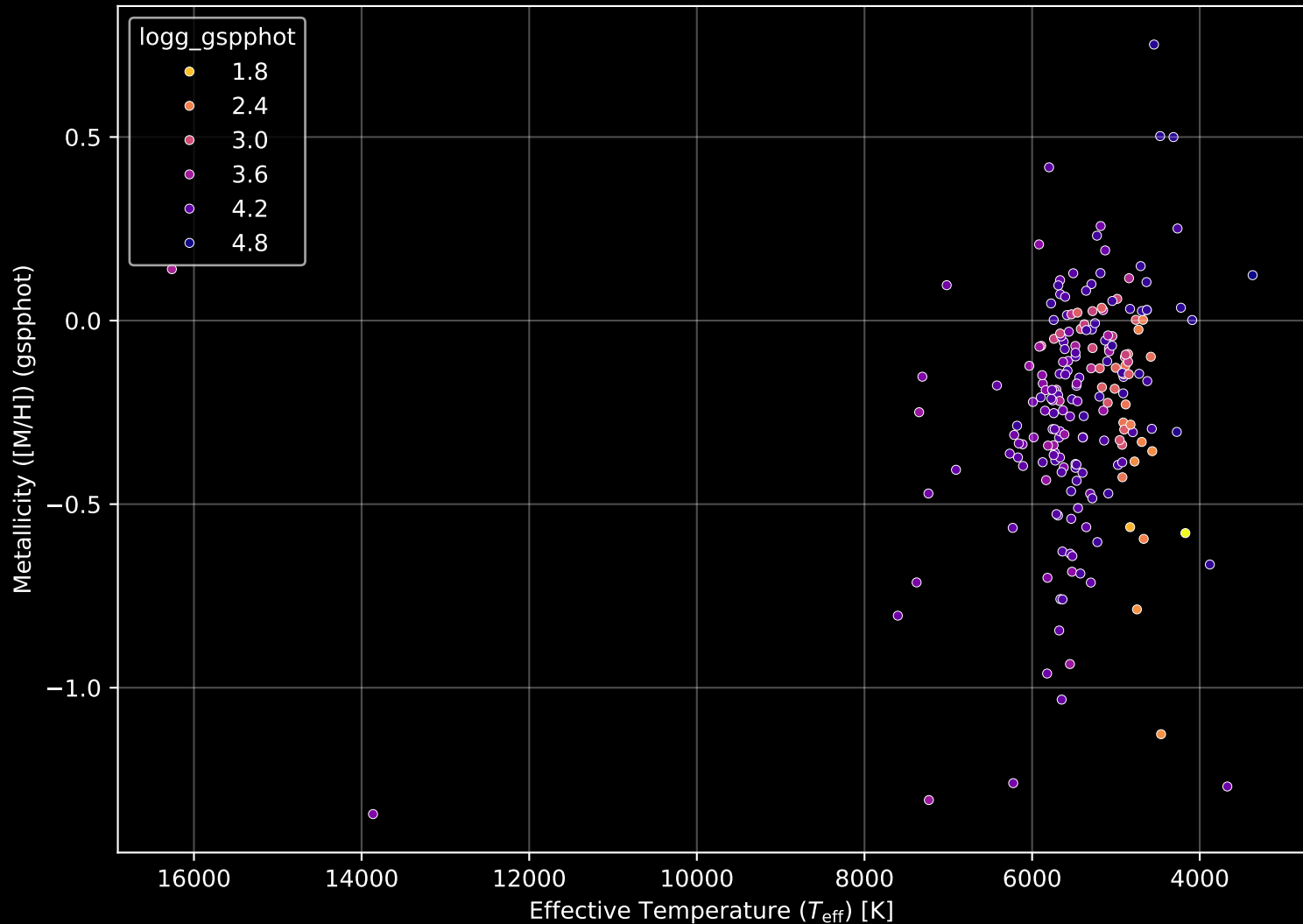
APOGEE DR17 Field: [090-30] Stellar Population Parameters (n= 202)
